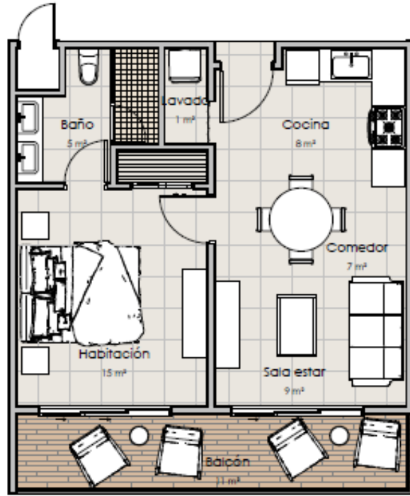
Apto. Tipo B 15 Und m2 Apto.: 51.5 m2 Balcón: 11 m2 Totales: 62.5
