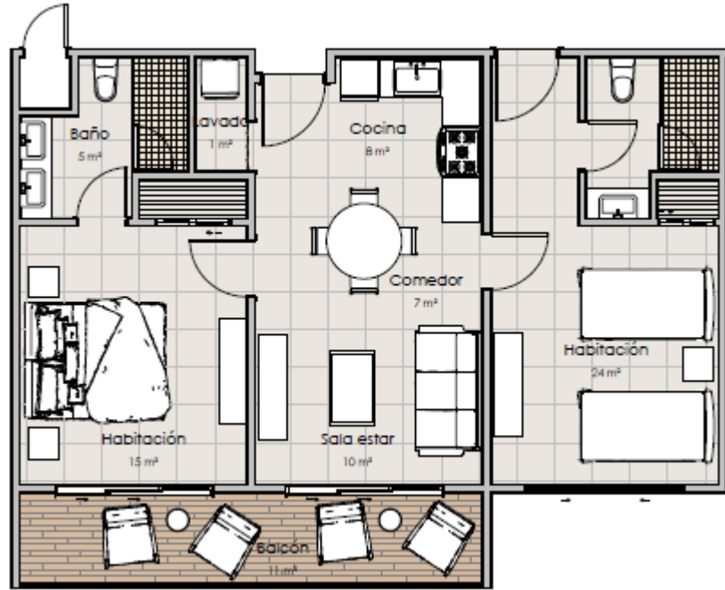
Apto. Tipo C 10 Und m2 Apto.: 84 m2 Balcón: 11 m2 Totales: 95
