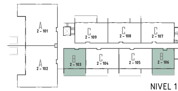
Apto. Tipo B 4 Und m2 Apto.: 51.5 m2 Balcón: 11 m2 Totales: 62.5
