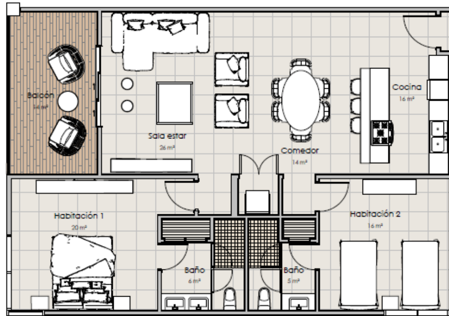
Apto. Tipo E 2 Und m2 Apto.: 116 m2 Balcón: 14 m2 Totales: 130
