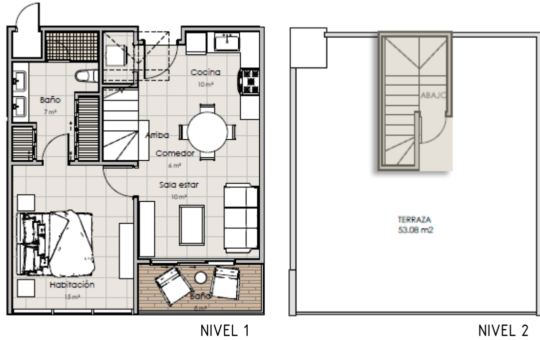
Apto. Tipo B PH 5 Und
