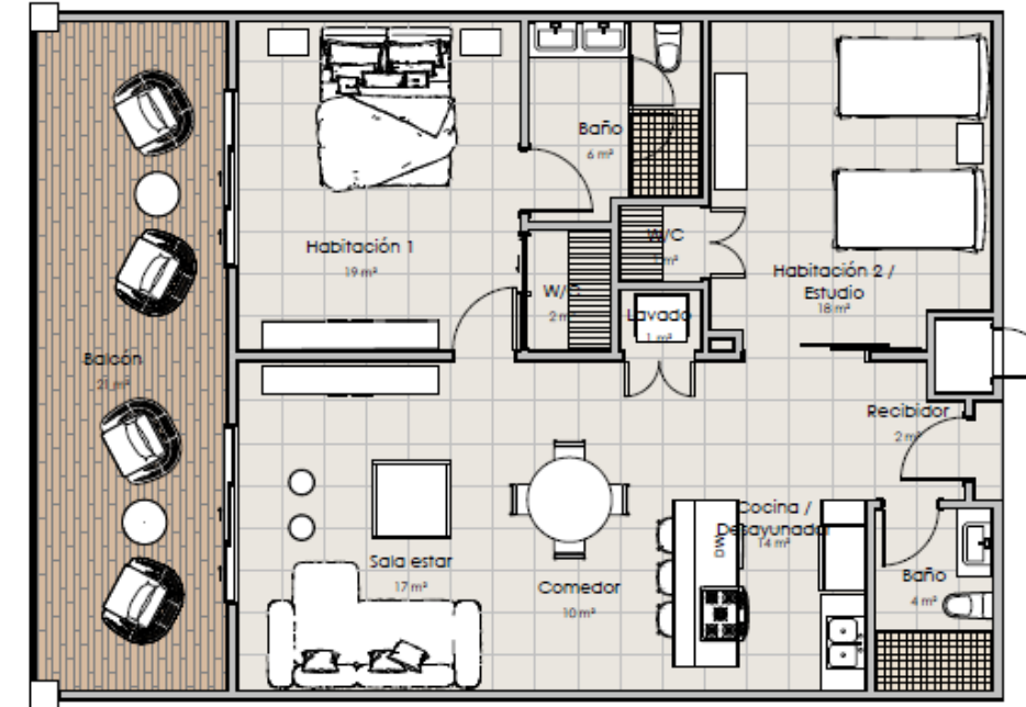
Apto. Tipo F 1 Und m2 Apto.: 116 m2 Balcón: 14 m2 Totales: 130
