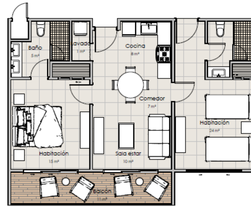
Apto. Tipo C 12 Und m2 Apto.: 84 m2 Balcón: 11 m2 Totales: 95
