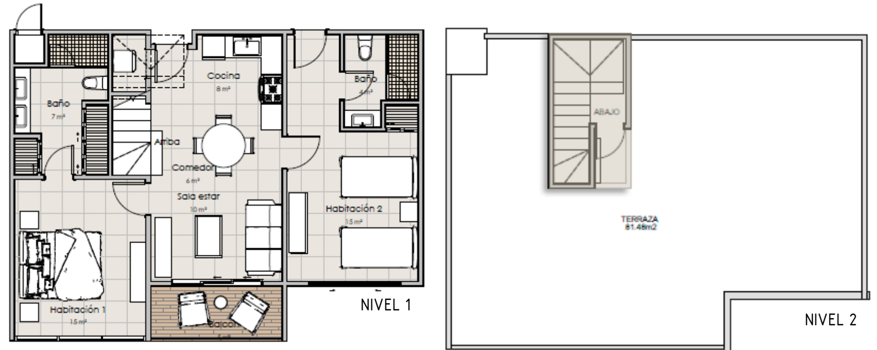
Apto. Tipo C PH 6 Und
