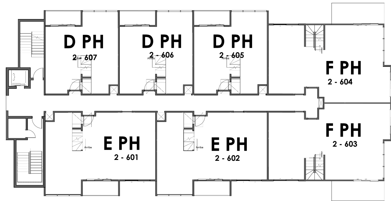
NIVEL 6 (PH)
