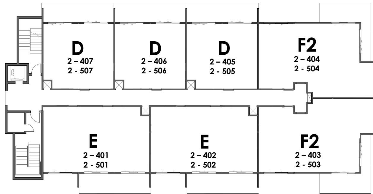
NIVELES 4 y 5
